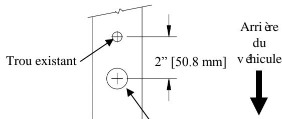
Figure 2 1" dia. – Percer Perçage des trous d'accès
